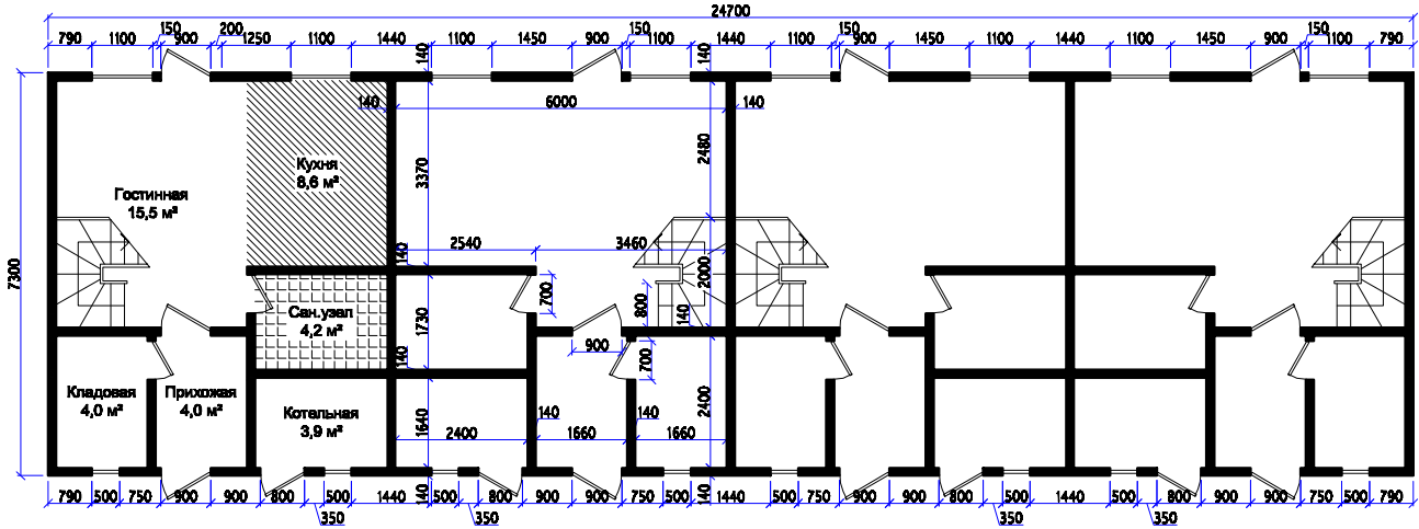
План 1го этажа
